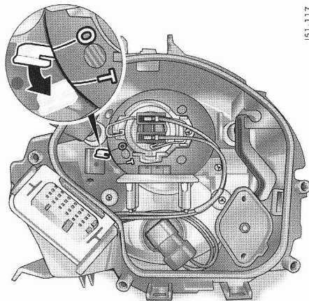
Projecteurs halogène
