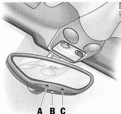
A - Capteur B - Interrupteur de réglage anti-éblouissement C - Diode lumineuse
