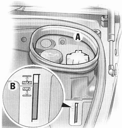
A - Bouchon du vase d'expansion B - Niveau de liquide de refroidissement
