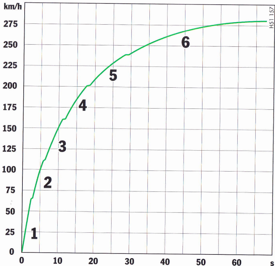
Diagramme d'accélération 911 Carrera, 911 Carrera 4, 911 Targa 4 à boîte mécanique (Les valeurs sont communiquées pour un poids à vide selon la norme DIN et avec demi-charge, sans équipement supplémentaire.)
