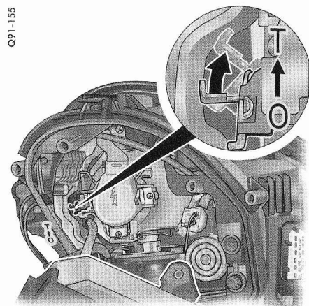
Projecteurs bi-xénon
