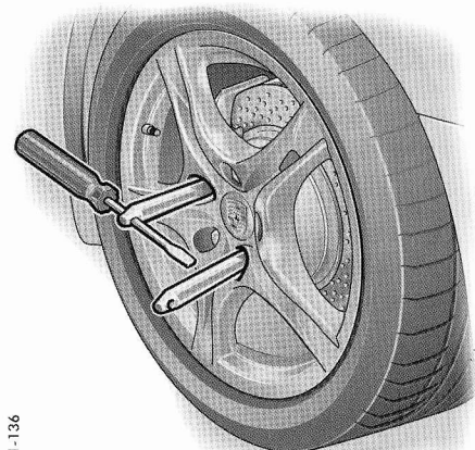
Vissage de 2 auxiliaires de montage sur les véhicules avec PCCB
