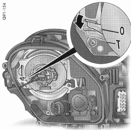
Phares halogène
