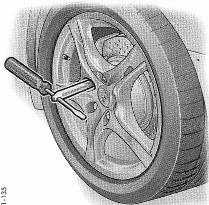
Vissage de l'auxiliaire de montage sur les véhicules sans PCCB
